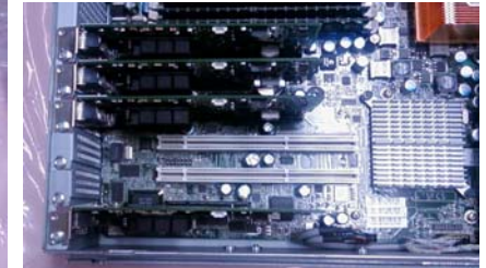
Infiniband ConnectX x 4 (各PCI-Express x 8lane)
